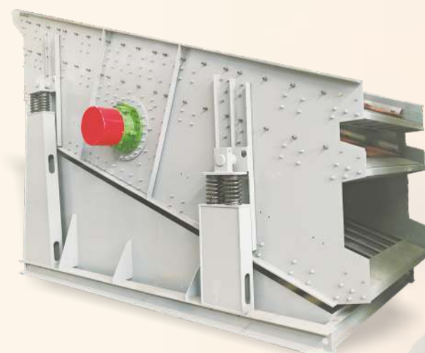
圆振筛 Круглый вибрационный грохот
